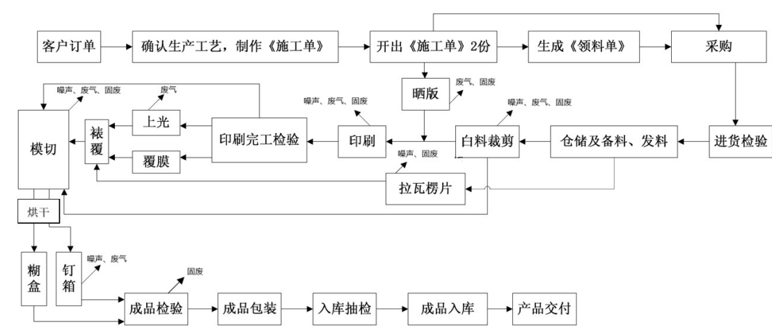
纸箱、纸盒生产工艺
